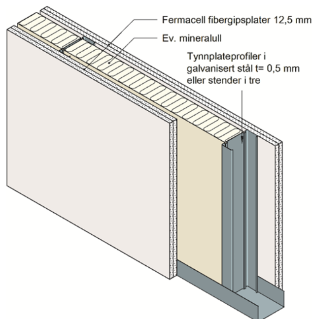
Fig. 1 Prinsipiell oppbygning av Fermacell Skilleveggsystem med stålprofiler
