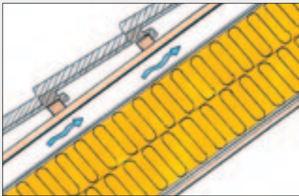
Prinsskisse ventilert takkonstruksjon
