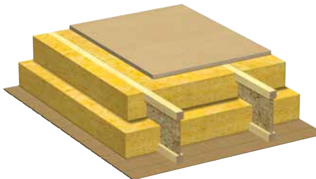
Fig. 1 Lydbjelkelag Masonite gulvbjelker fullisolert med himling festet rett til gulvbjelkene. 1)
