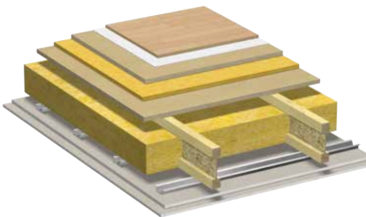
Fig. 7 Lydbjelkelag Masonite gulvbjelker med himling av to platelag, se oppbygging.
