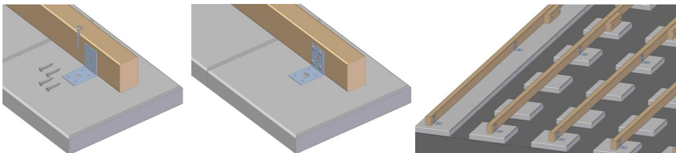
Festing av terrassebordene
